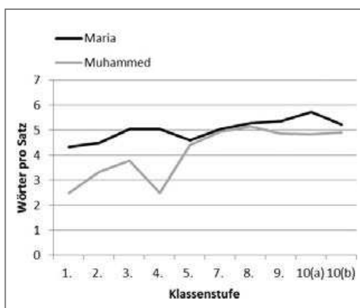
Abb. 6 : Mittlere Satzlänge
