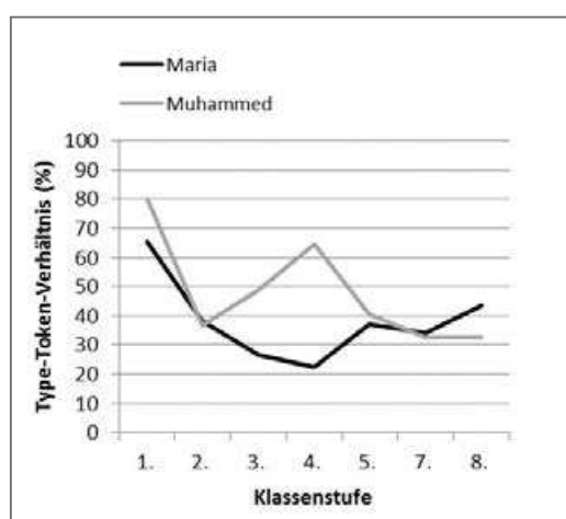
Abb. 4: Type-Token-Verhältnis
